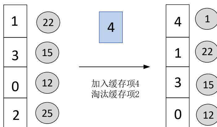
图4.8 LRU 缓存污染问题
