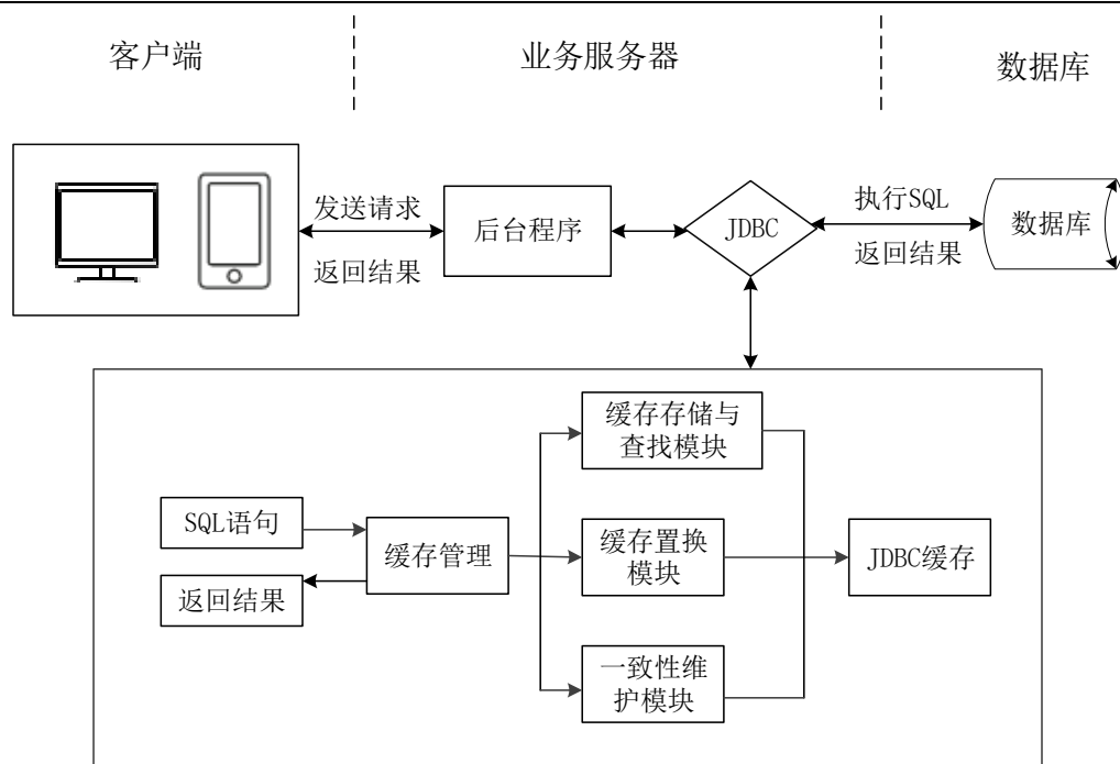
图4.4 JDBC 缓存数据管理模型
