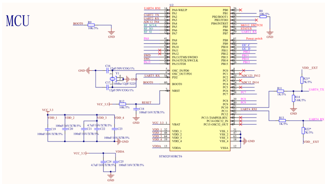
图2.3 MCU 原理图
