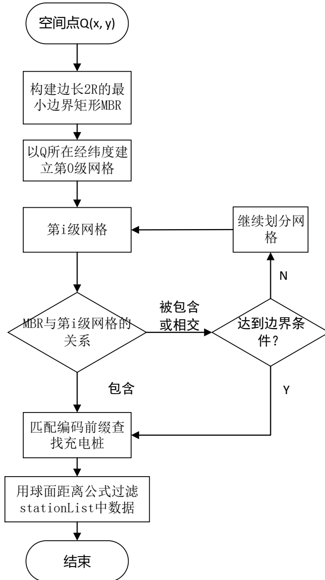
图3.10 查找算法流程
